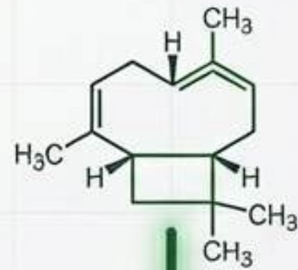
Molécula Beta-Caryophyllene
